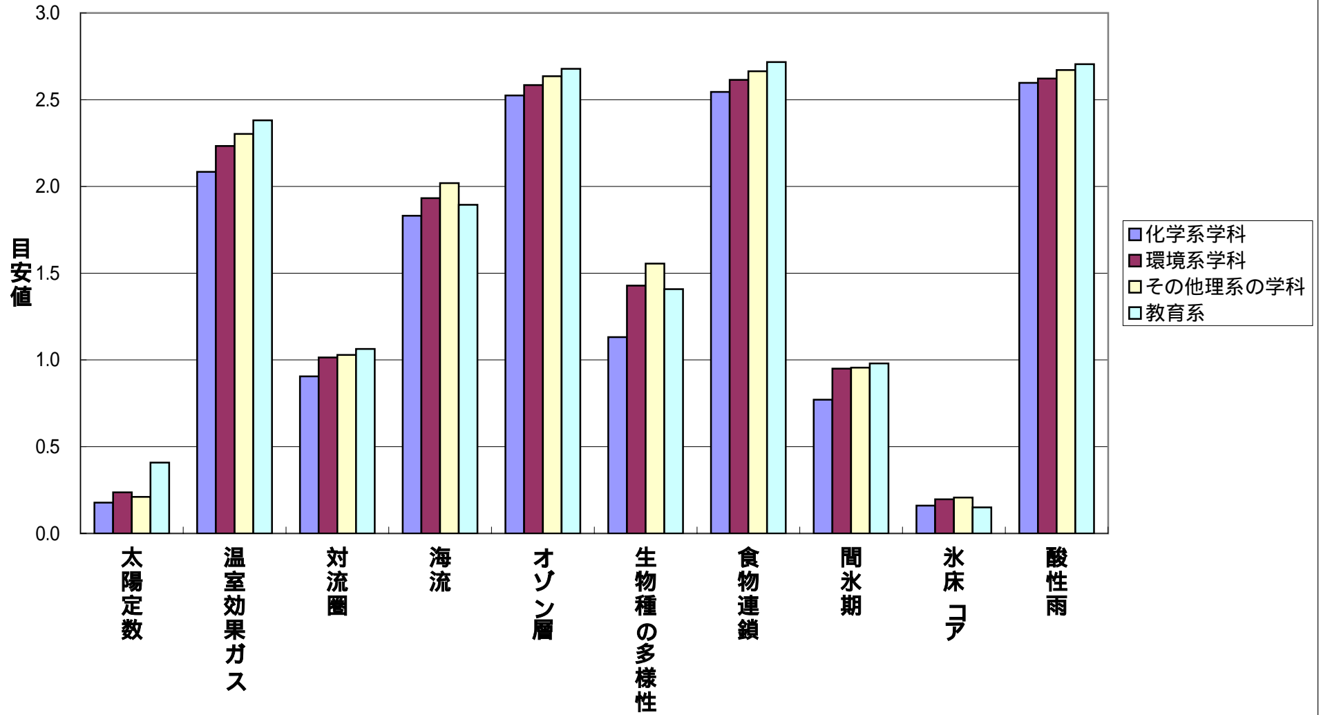
図2 地球環境
