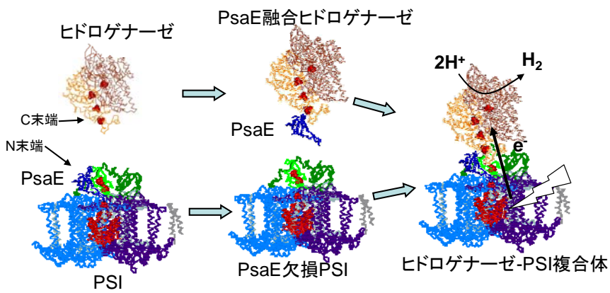
図7 ヒドロゲナーゼ-PSI 複合体の設計
