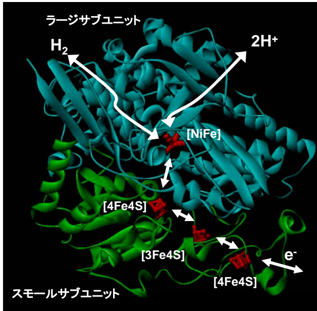
図3 [NiFe]ヒドロゲナーゼの構造
