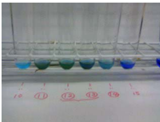
図 1 数字はギ酸 1 滴に対するフェーリング液の滴数
