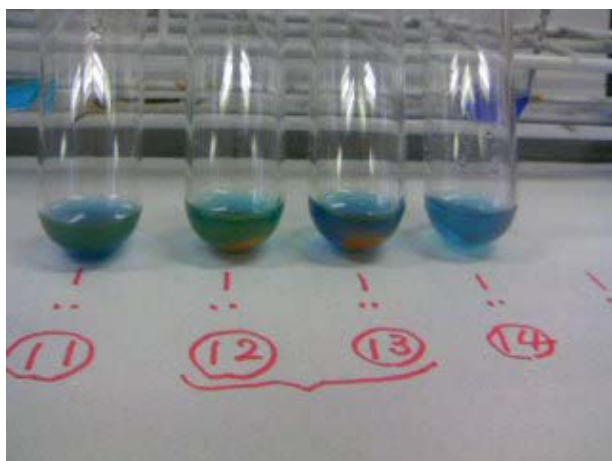
図 2 赤色に見えるのが、酸化銅 (I) <color>
