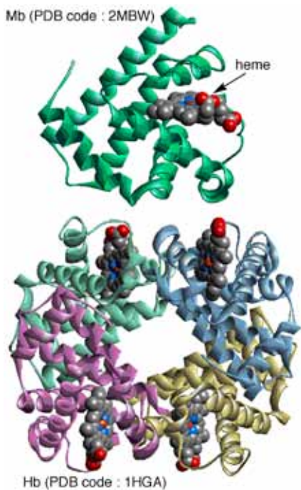
図1 ヘモグロビンとミオグロビンの構造
