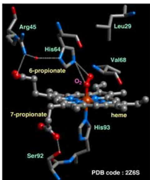
図2 マッコウジラミオグロビン内での酸素錯体構造
