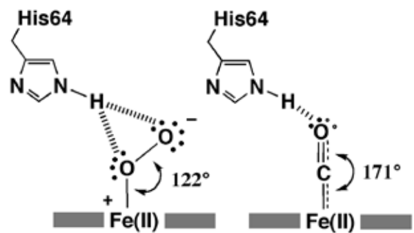
図3 リガンド( O_2 , CO)選択性に関する説明
