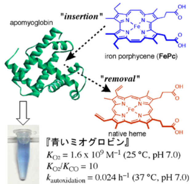
図4 スーパーミオグロビンをめざして
