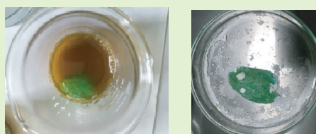
■左：飽和溶液中の結晶， 右：3カ月放置後（P17，写真4）
