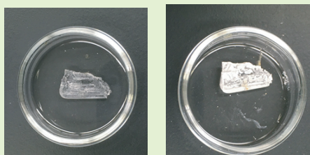
■左：溶液から引き上げた直後， 右：空気を抜いた後（P17，写真2）
