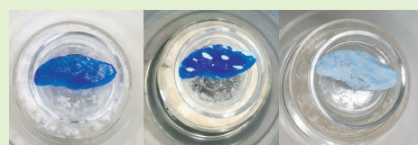
■左：0日目，中央：7日後，右：14日後 （P17，写真5）
