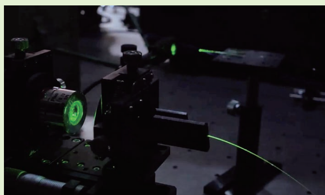
■ 通信用光ファイバーに緑色 (波長 532 nm) のレーザー光を伝搬させているデモンストレーション実験 (P250, 図 3)
