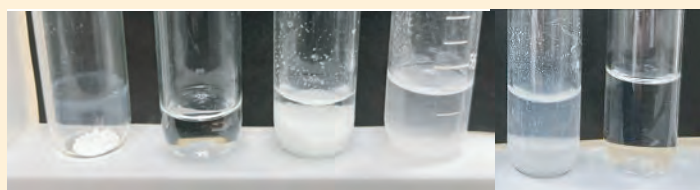
■ \text{Pb}^{2+} の検出 (P107, 写真 1)
