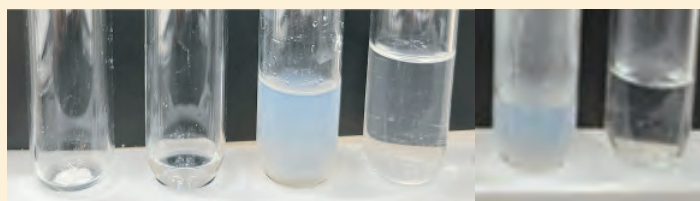
■ \text{Zn}^{2+} の検出 (P107, 写真 2)
