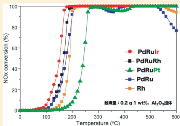
■ NO x 還元反応の転化率の温度依存性 (P350, 図 4)
